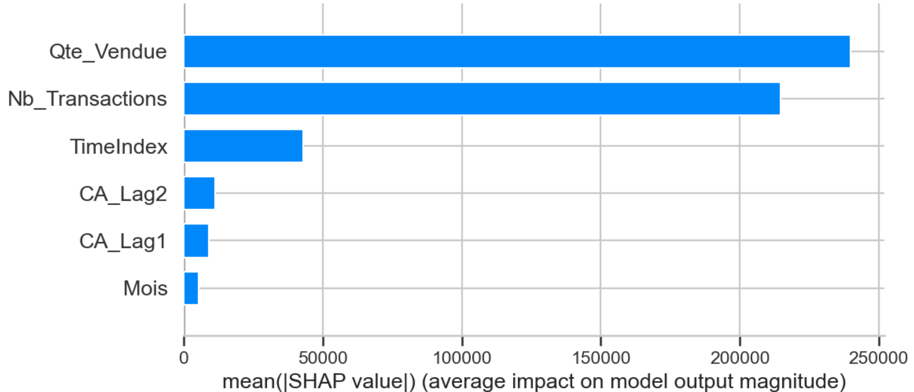
SHAP — Importance Globale des Variables
